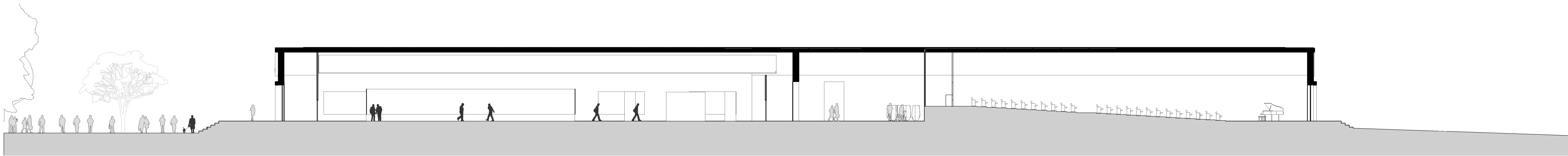
SEZIONE B_B 1:200
