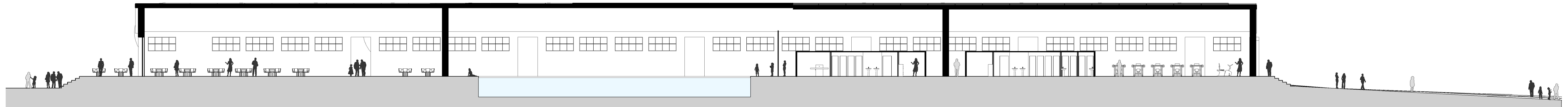
SEZIONE A_A 1:200
